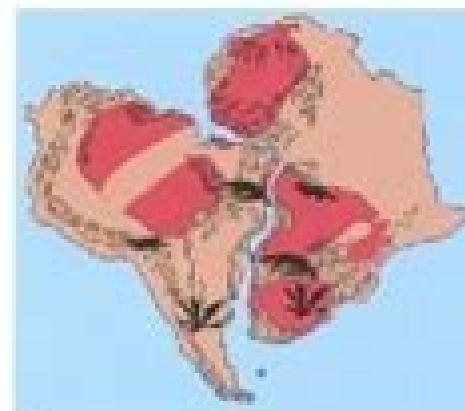
Fig. 10 - Les continents dérivent d'un bloc unique, les continents anciens, les continents nouveaux.
