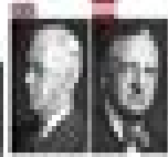
Cajal 1906 Golgi 1906
