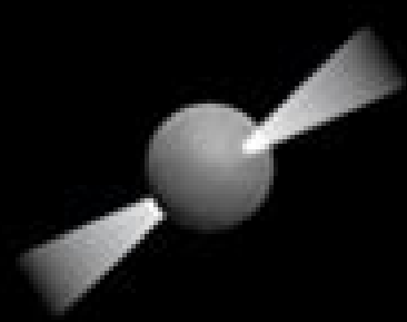
pulsars
