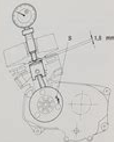
Fig. 21 (misura master cyl.)
