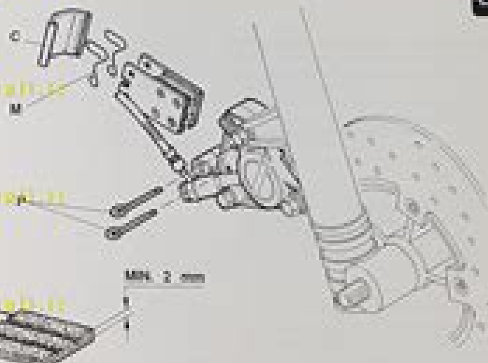
Fig. 23 (ispezione minimo pastiglie)
