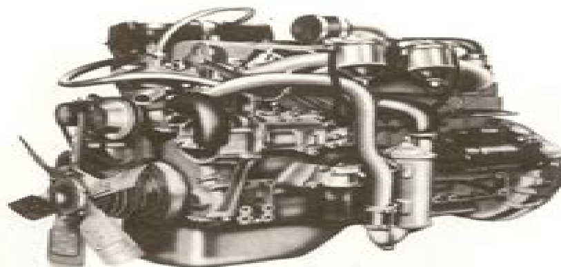
Motor 797-05 pentru autocamioane, autobasculante, autotractoare și autogăsiuni tip ROMAN 8.135 și 12.135
