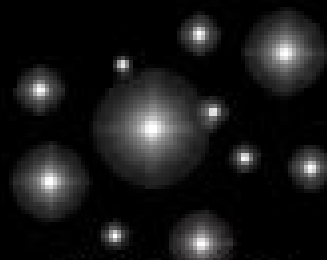
amas stellaires
