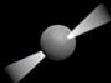
pulsars
