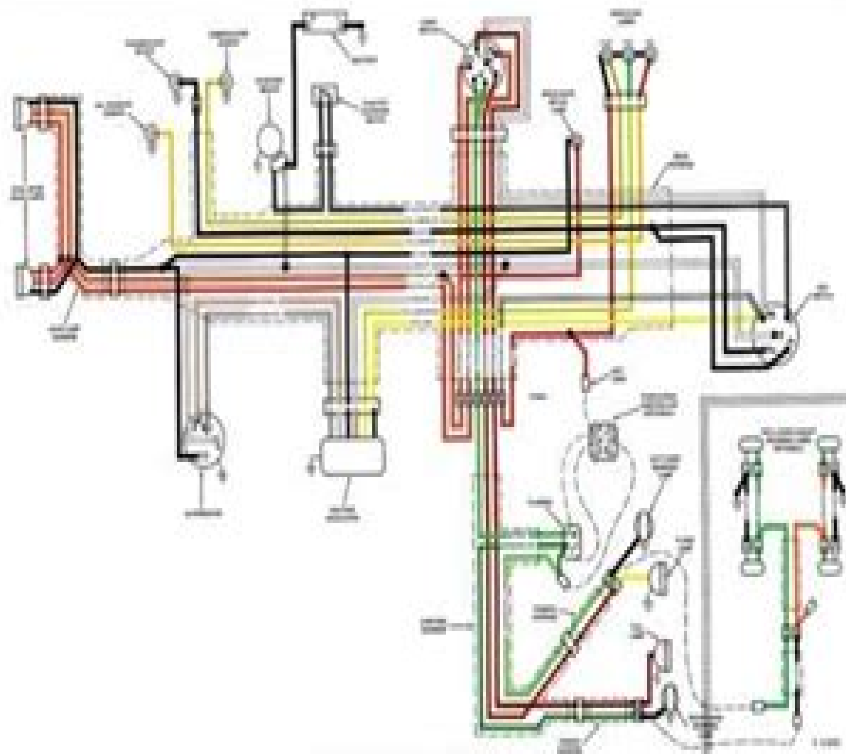
Fig. 1 Power Wiring (2007-2008) (2009-2010) (2011-2012)
