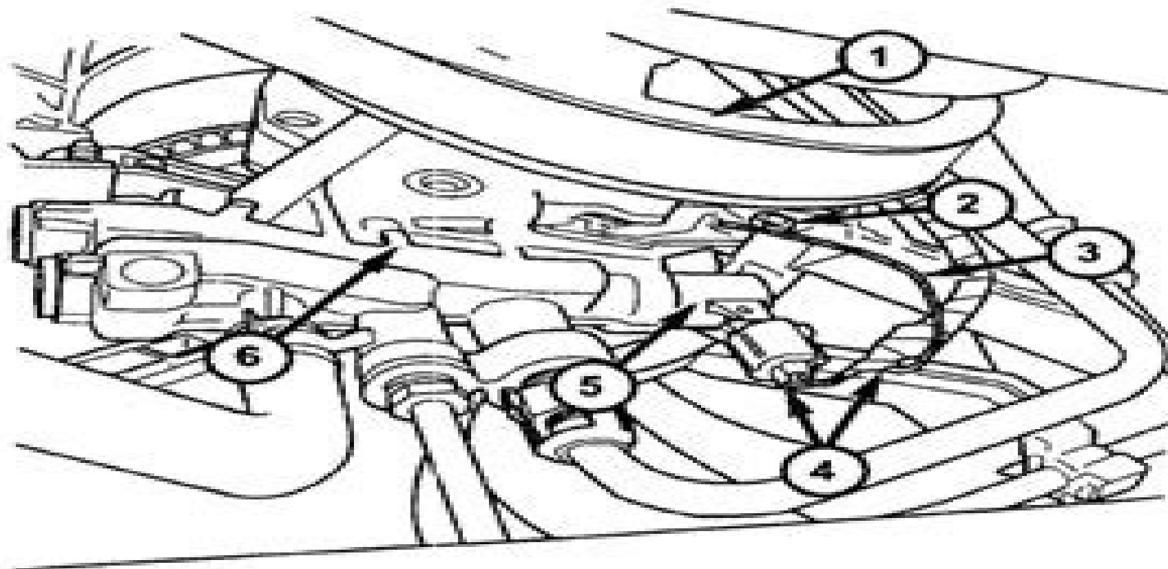
Fig. 1 HYDRAULIC FAN MODULE / SOLENOID
