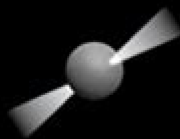
pulsars
