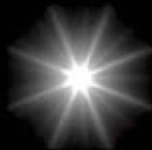
quasars
