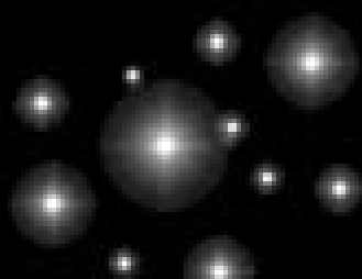
amas stellaires
