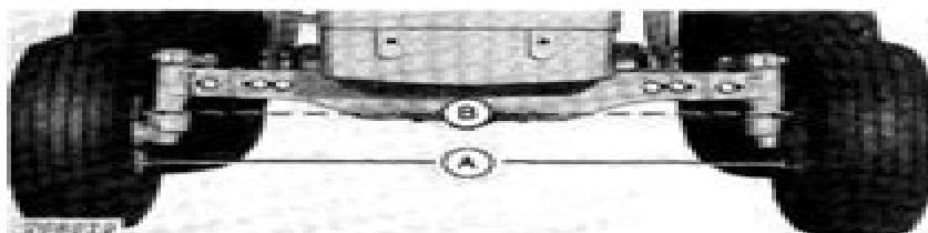
Fig. 31—Checking Toe-In
