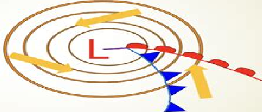
(d) Mature (initial occlusion)
