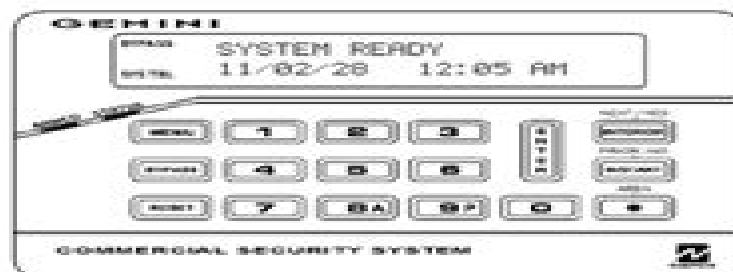
GEMC-BK1 Keypad
