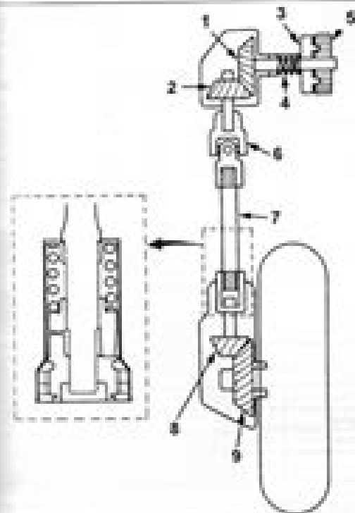
Principio de transmisión secundaria por cardán.
