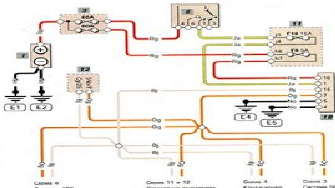
Диагностический разъем
