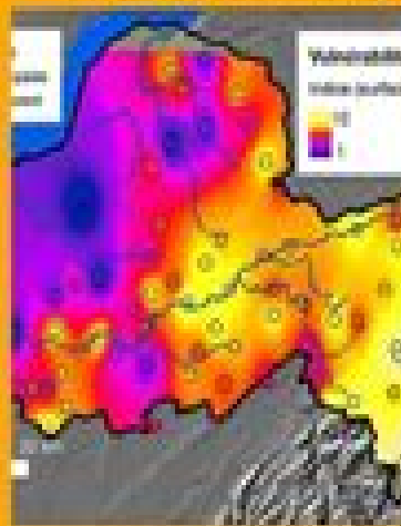
CARTE GÉOCHIMIQUE
