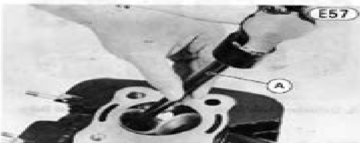
A. Valve Guide Arbor (57001-163)
