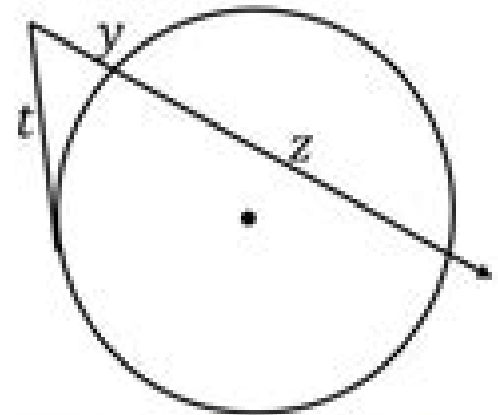
Tangent & Secant
