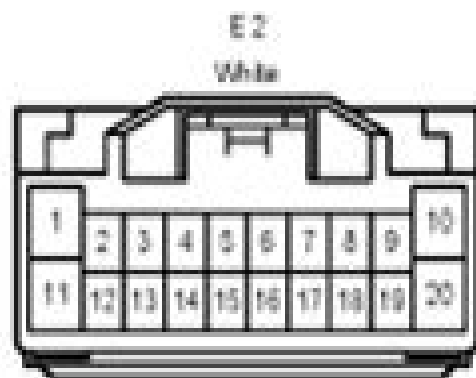
E2 Connector
