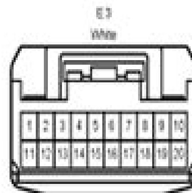
E3 Connector
