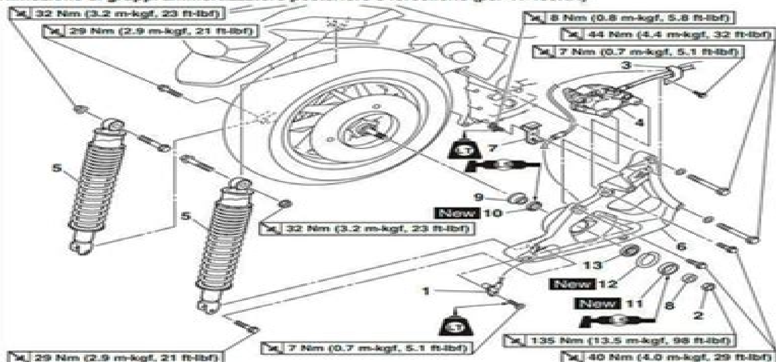
Rimozione di gruppi ammortizzatore posteriore e forcellone (per YP400RA)
