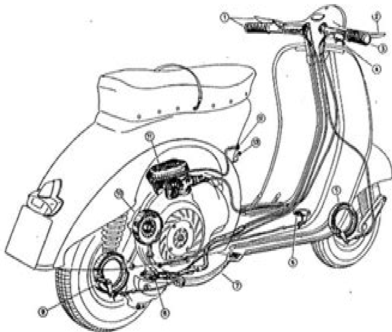
Fig. 6.—Instalación de mandos y transmisiones.
