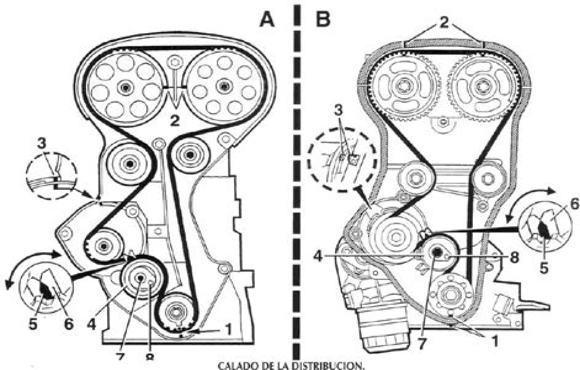
A. Motor 1.6 - B. Motores 1.8 y 2.0 - 1. Marca de rueda dentada de cigüeñal - 2. Marcas de ruedas dentadas de ejes de levas - 3. Marca de bomba de agua - 4. Rodillo tensor - 5. Indicador de rodillo tensor - 6. Muesca de rodillo tensor - 7. Fijación del rodillo tensor - 8. Hueco hexagonal de reglaje.
