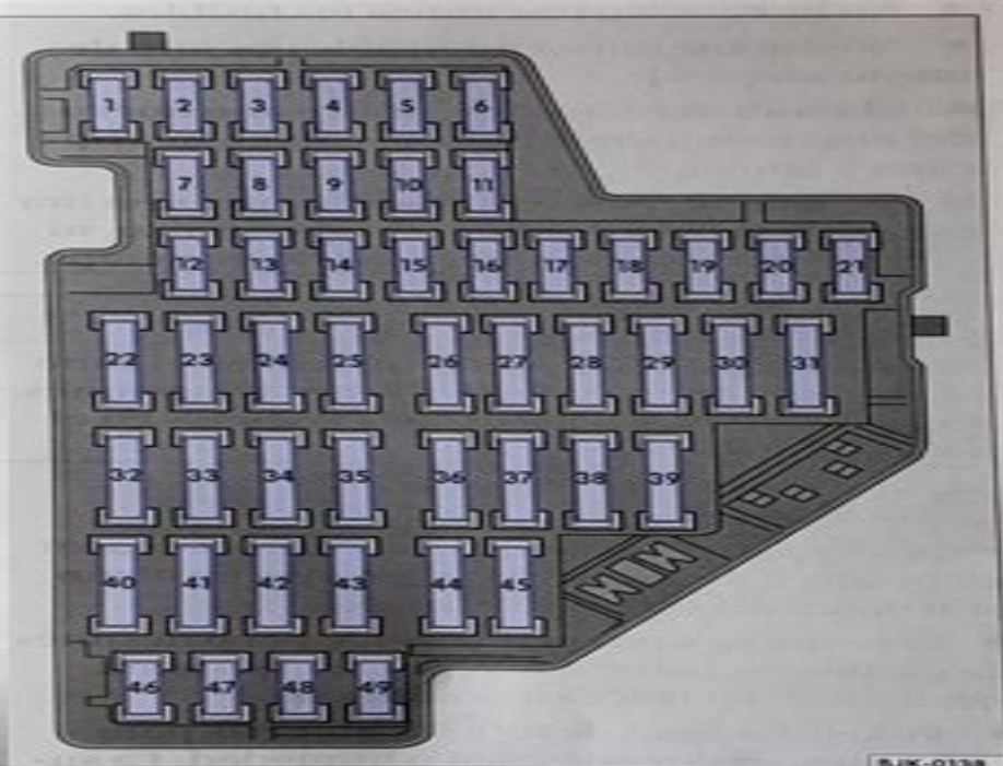
Fig. 205 Cajas de fusibles del tablero de instrumentos
