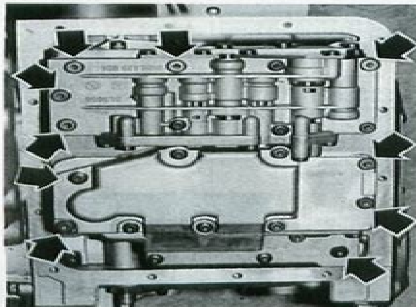
Situación de los 10 tornillos de fijación del bloque hidráulico
