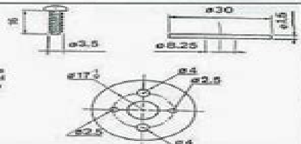
Cotas de fabricación de la arandela de extracción del retén de eje de selección
