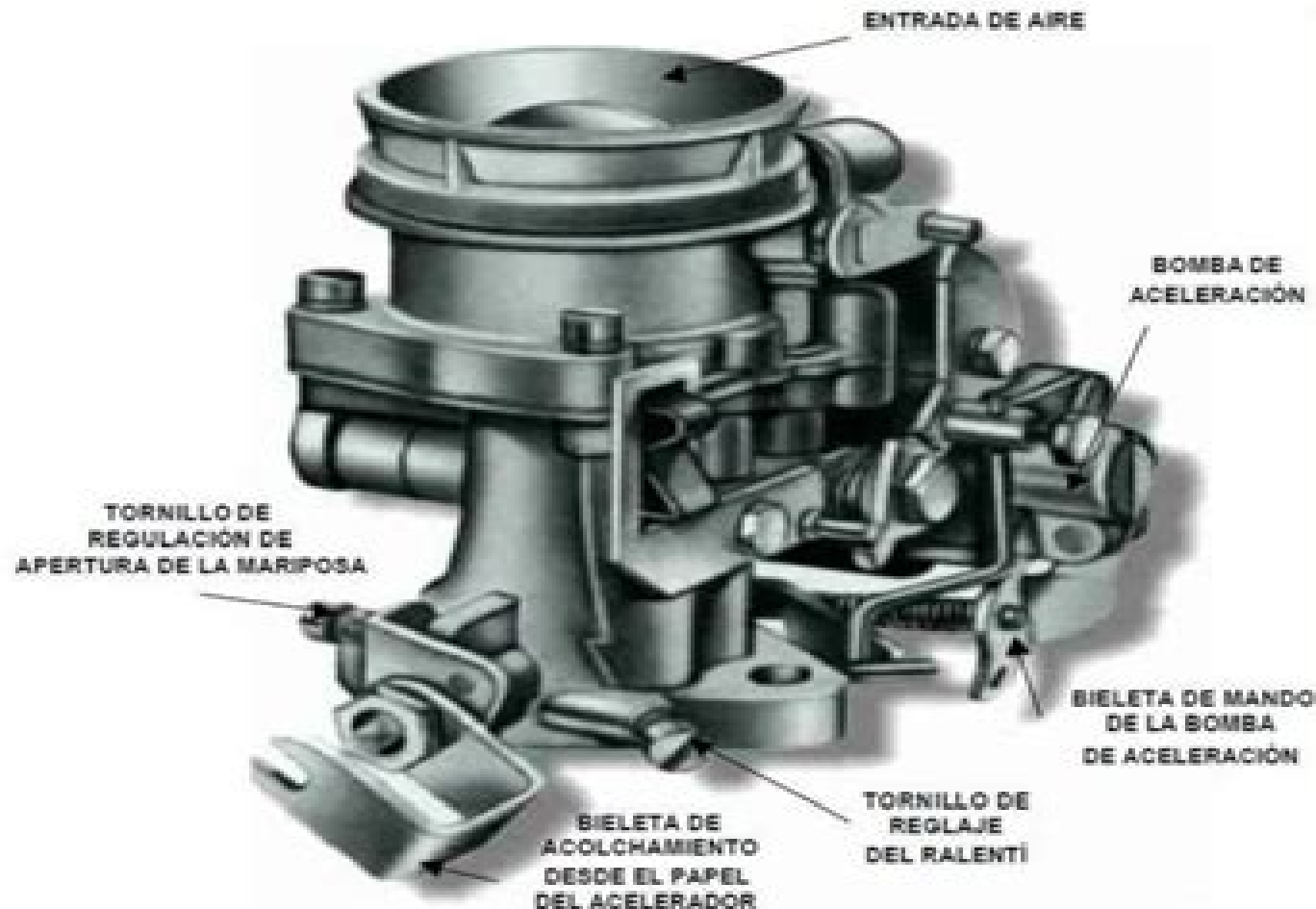
CARBURADOR
