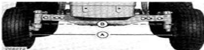
Fig. 31—Checking Toe-In
