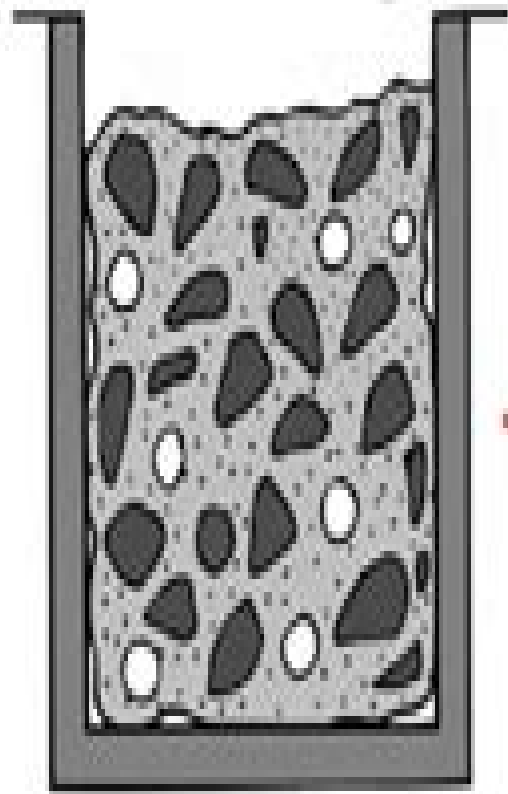
Béton coulé en plein
