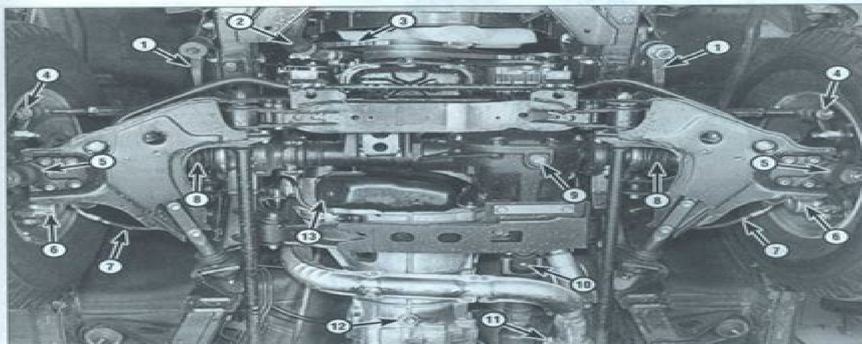
Vista inferior del motor/transmisión V6 - 4WD (típico)
