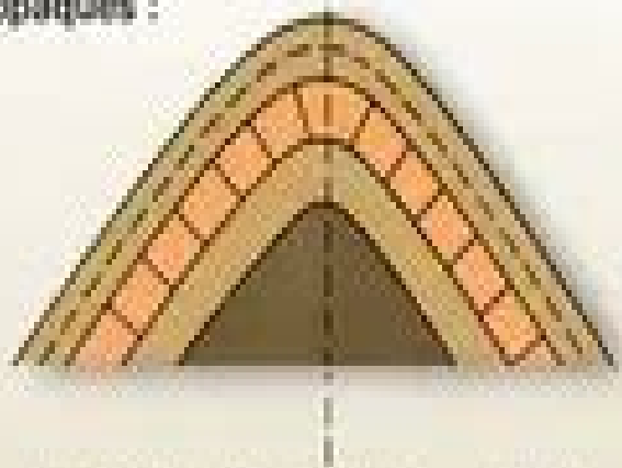
droit : le plan axial est vertical
