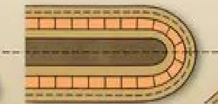
couché : les deux flancs et le plan axial sont horizontaux
