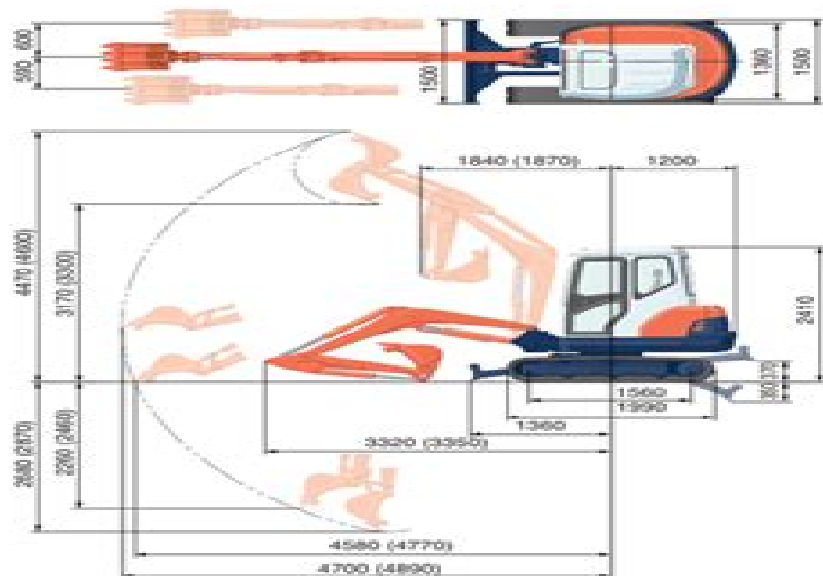
①: Long Arm Unit, mm
