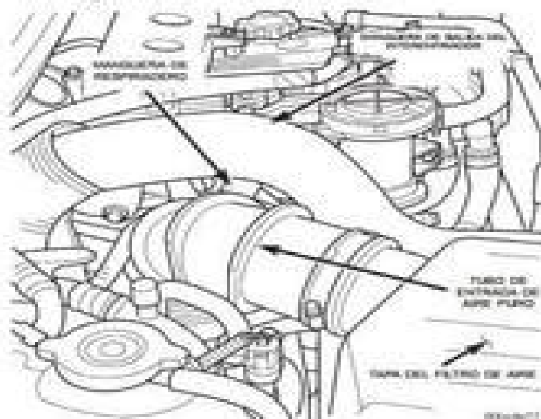
Fig. 2 Mangueras de admisión de aire
