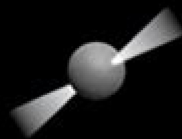
pulsars
