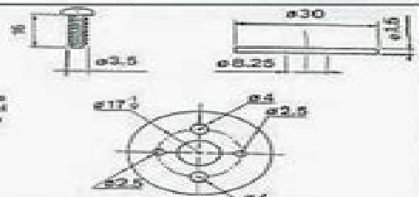
Cotas de fabricación de la arandela de extracción del retén del eje de selección
