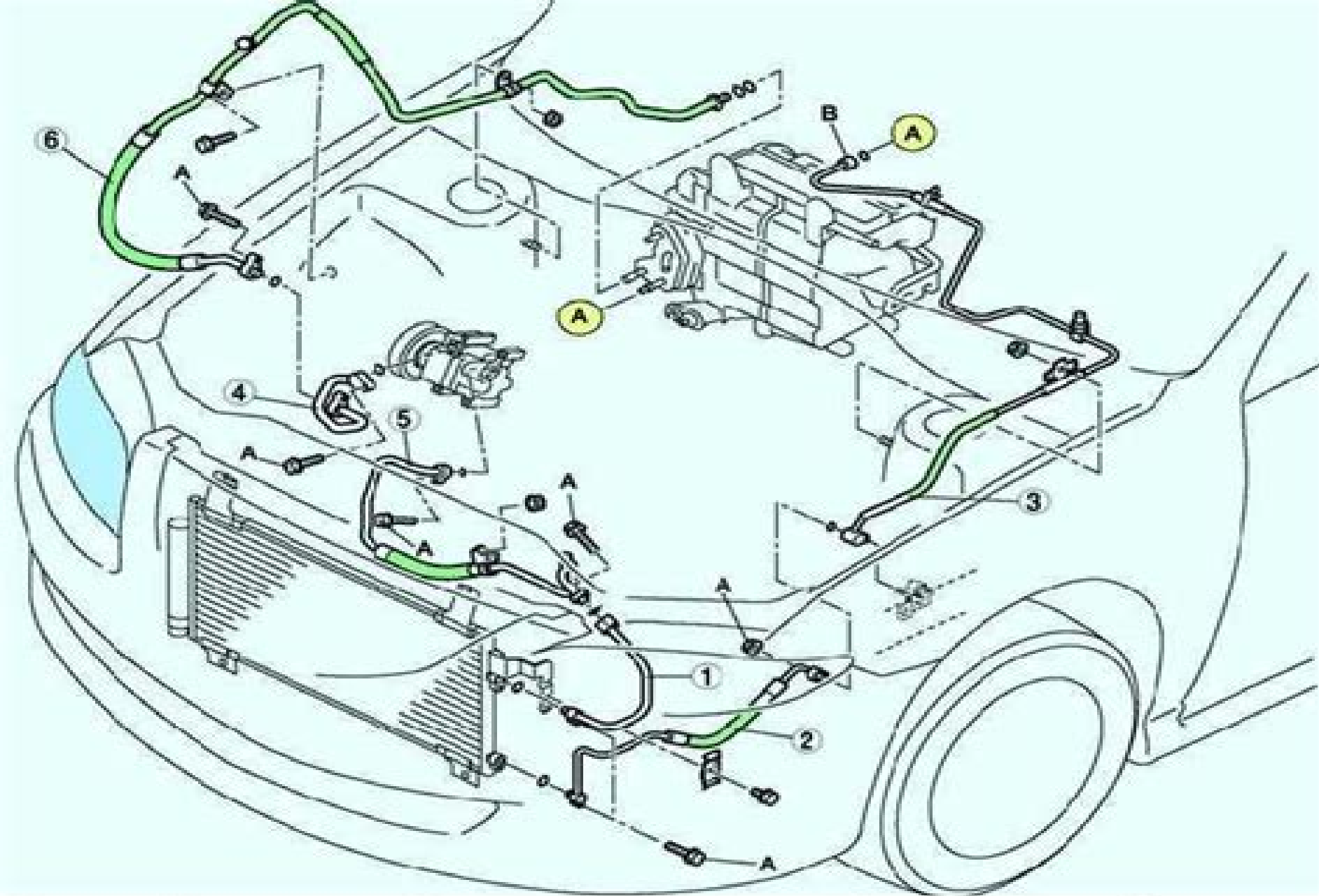
Линия хладагента автомобиля Mazda 3: 1 – трубка охладителя №1; 2 – трубка охладителя №2; 3 – трубка охладителя №3; 4 – трубка охладителя №4; 5 – шланг охладителя (верхний); 6 – шланг охладителя (нижний)
