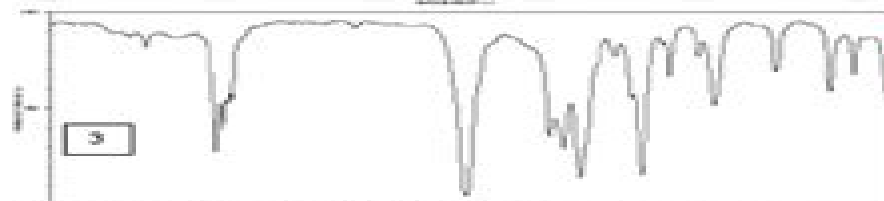
butanone
