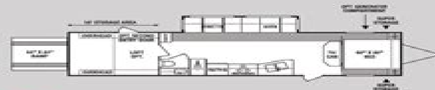
36P • UNW 8970 • Dry Hitch Wt. 910 • NCC 5030 • Length 37'8"
