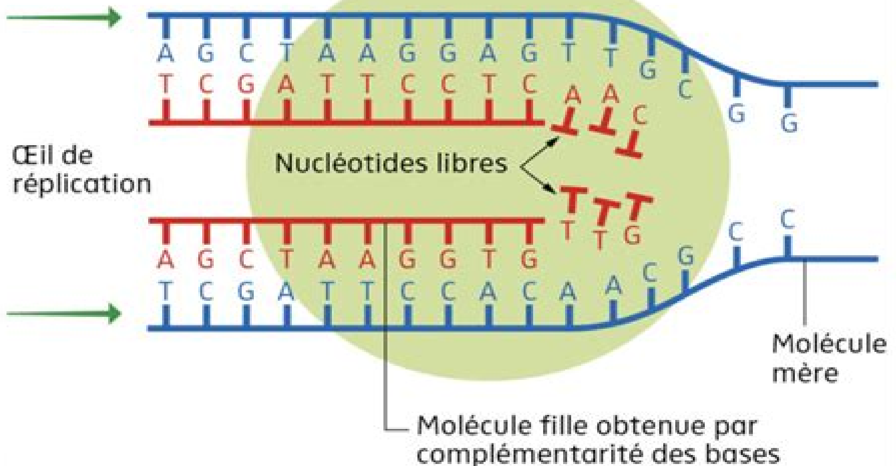
c Représentation simplifiée d'une fourche de réplication. Remarque : une seule ADN polymérase est ici représentée.
