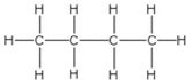
Butane
