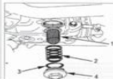
Montage de la tige de câble d'huile : 1. Tensionner 2. Ressort d'appui 3. Joint torique 4. Roulement
